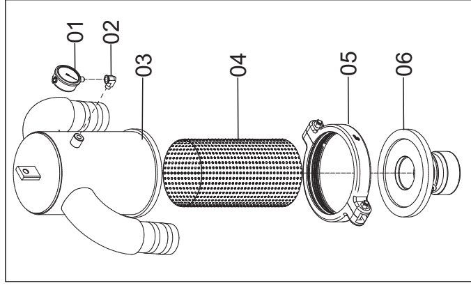
FILTRO APARTIR 10/2017
