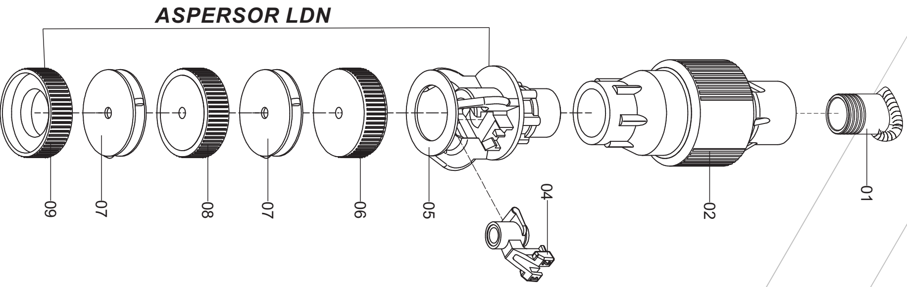
MOD. NOVO
