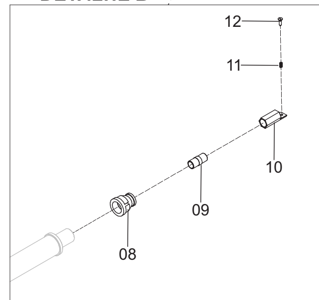
DETALHE B
