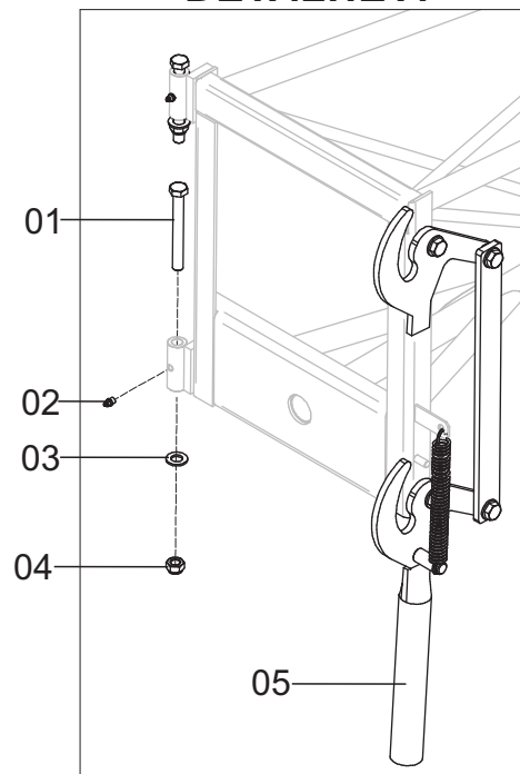
DETALHE A
